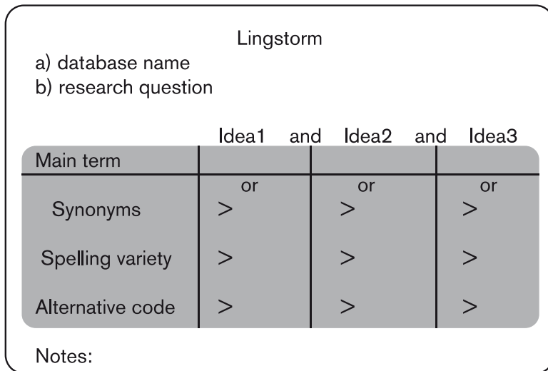
Fig. 3 Lluvia lingüística.
